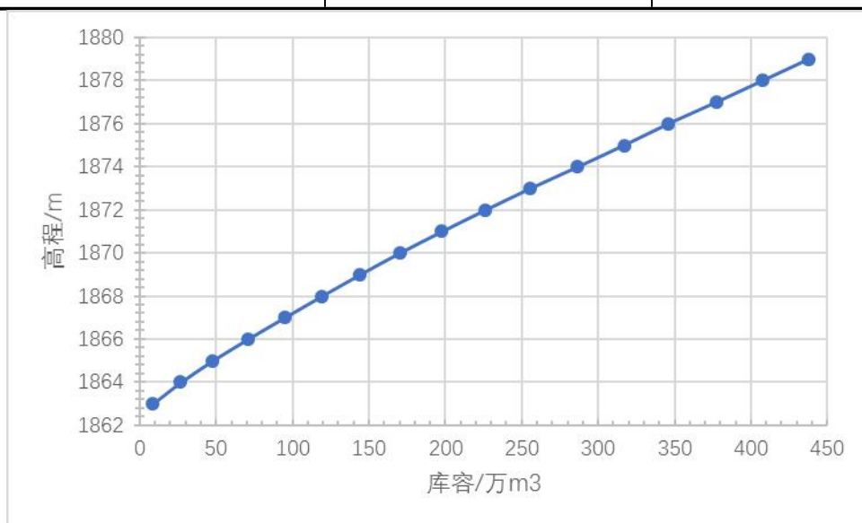
图 4.5-1 水库库容特性曲线图
