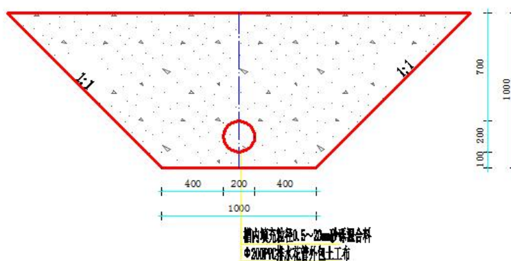
图 2-2 渗水防护结构图
