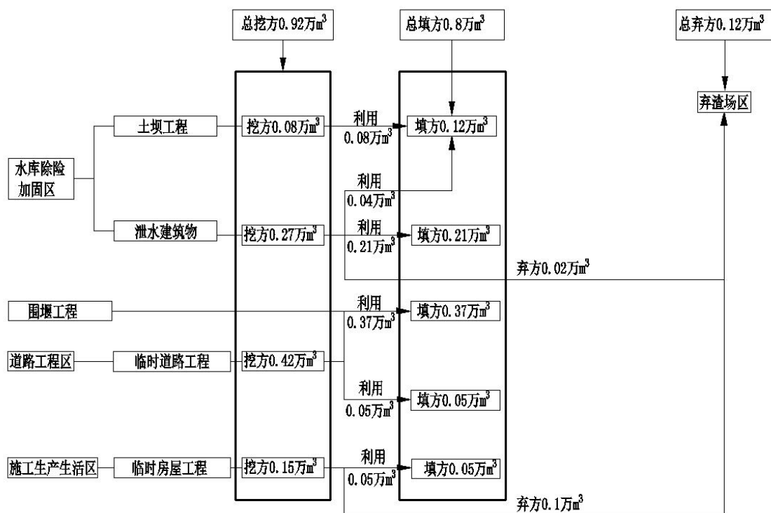
图 2-3 土石方流向框图
