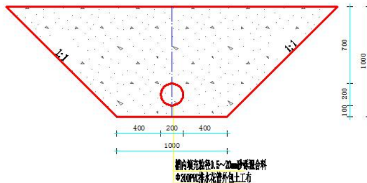
图 3.4-2 渗水防护结构图
