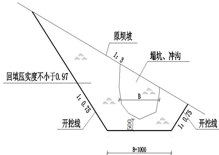
图 3.4-1 坝坡冲沟开挖回填示意图
