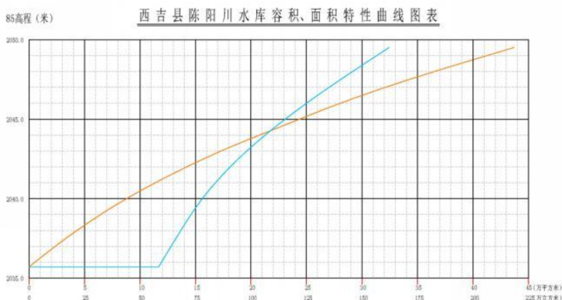
图5.2-1 水库水位~库容关系图
