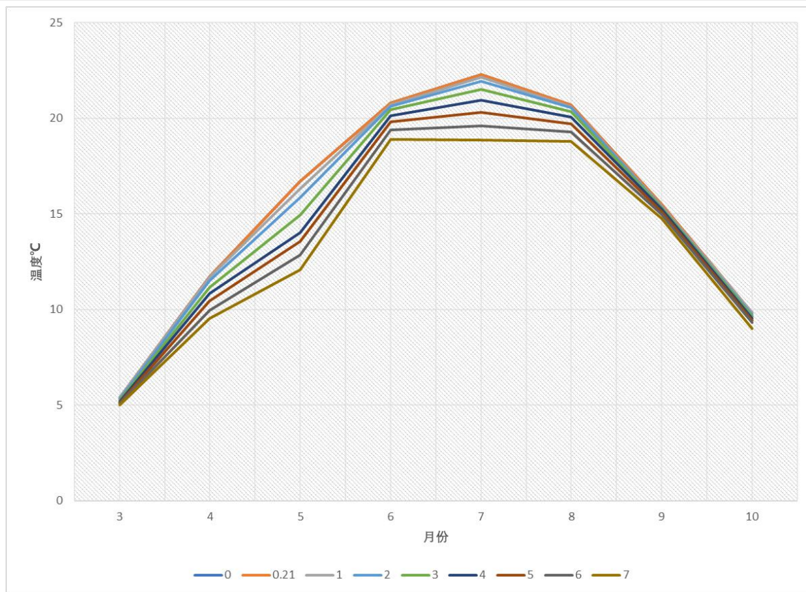
图5.2-1 地表水水温预测结果
